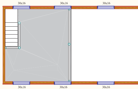
Loft Plan
