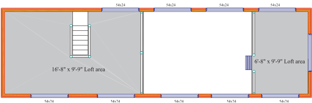
Loft Plan
