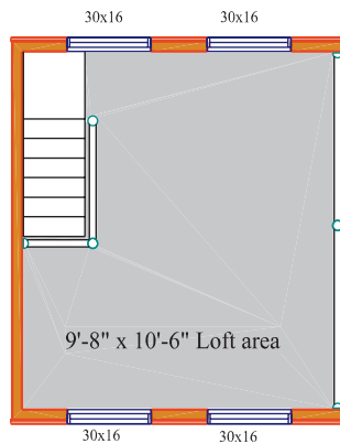
Loft Plan
