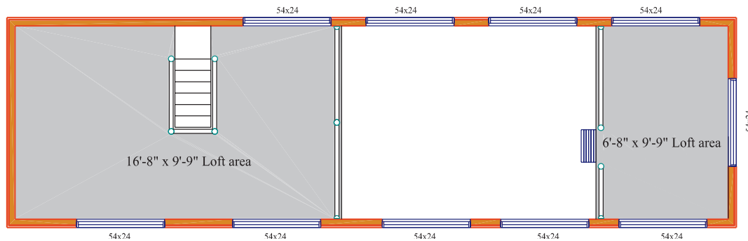
Loft Plan
