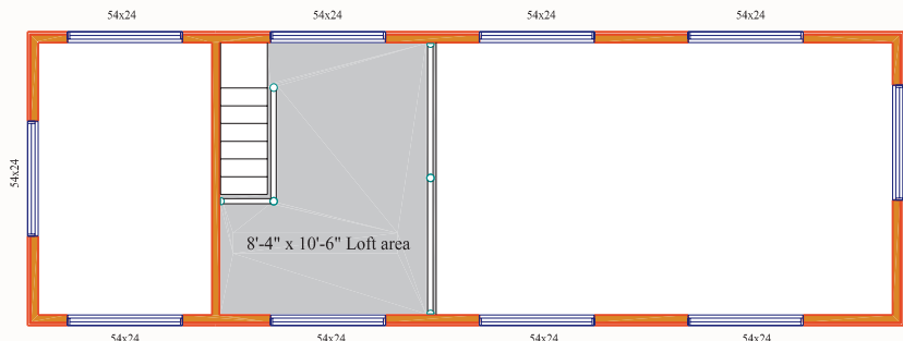
Loft Plan
